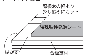
図2 ジーキャッチ裏面
