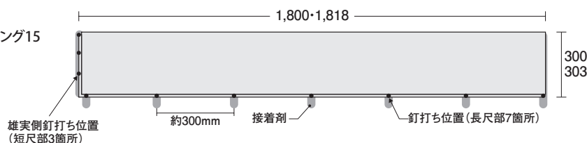
図3 (単位:mm)
