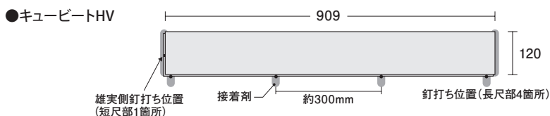
図3(単位:mm)
